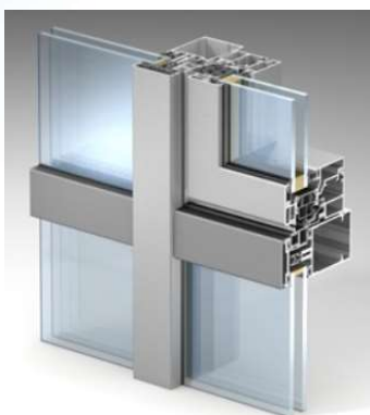
MODULOVÁ FASÁDA
