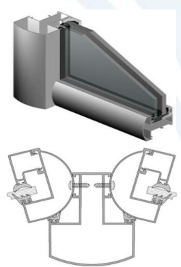
ODVETRANÁ FASÁDA
